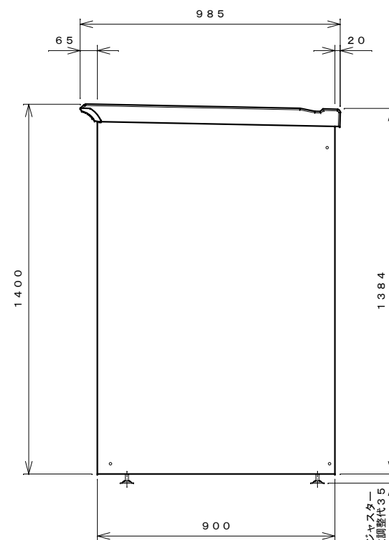
右側面図
