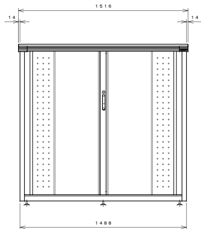
正面図
