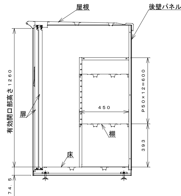
側面断面図
