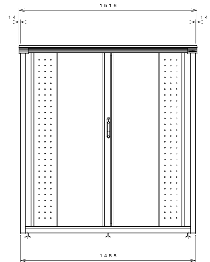
正面図
