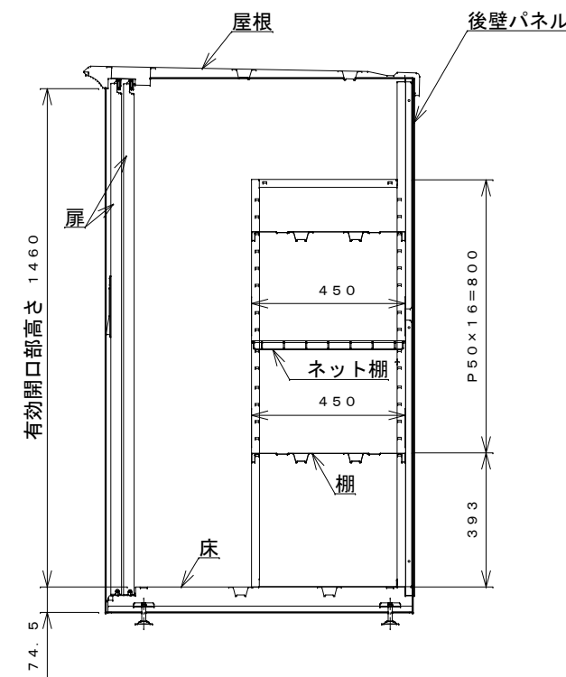
側面断面図
