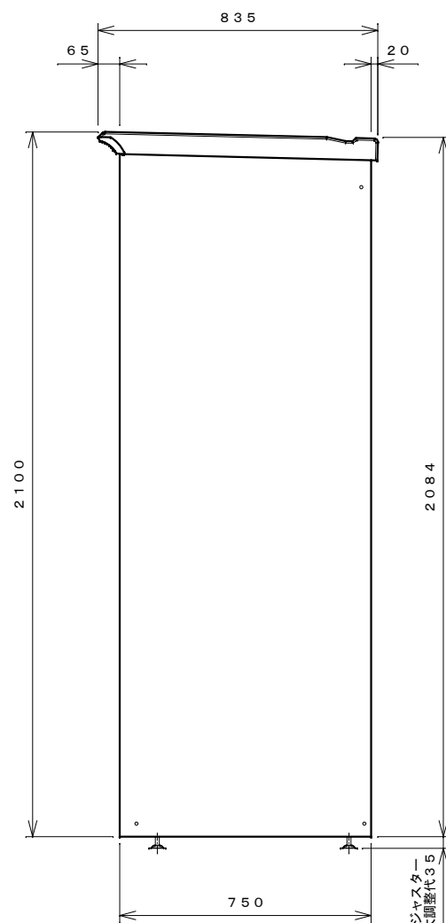
右側面図
