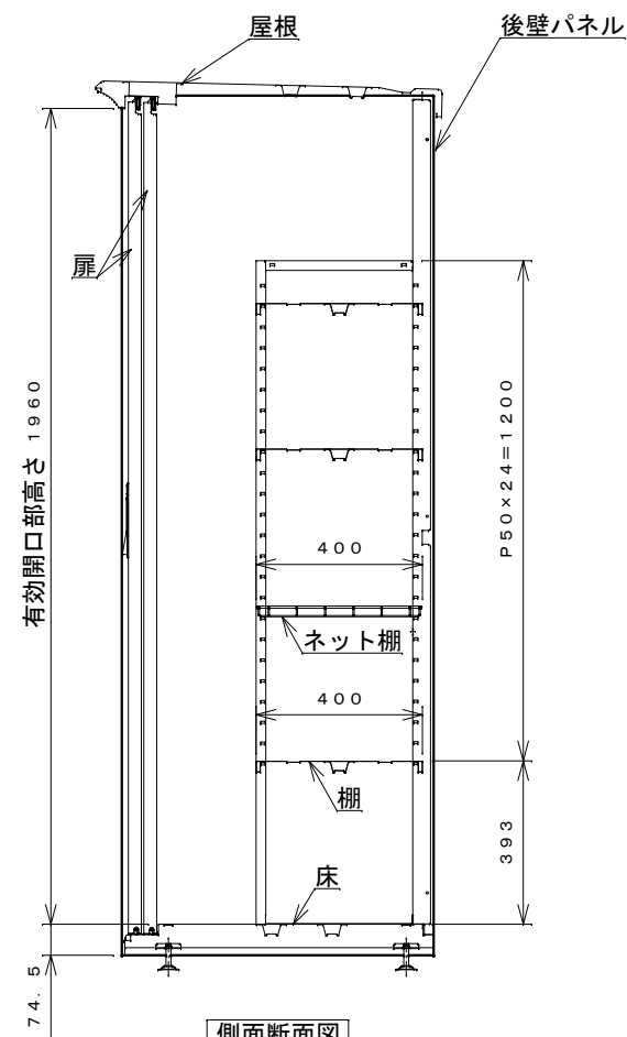
側面断面図
