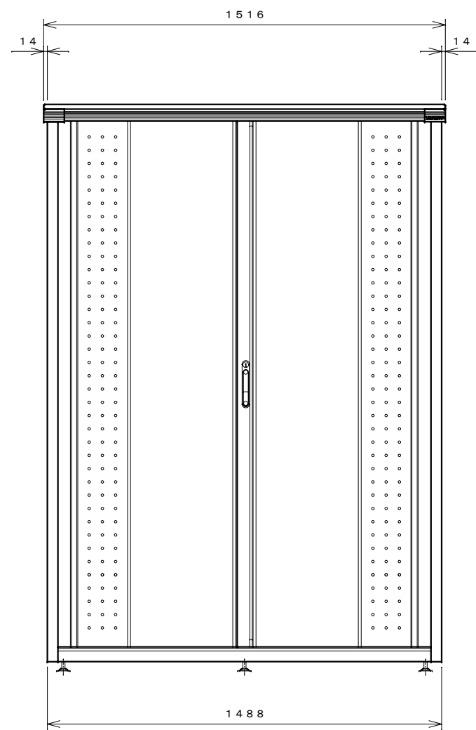
正面図
