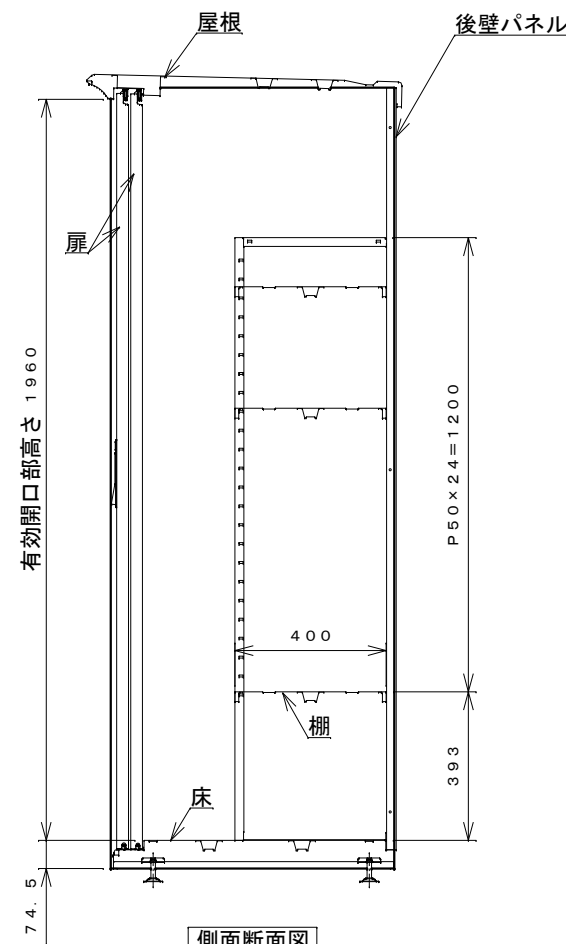
側面断面図
