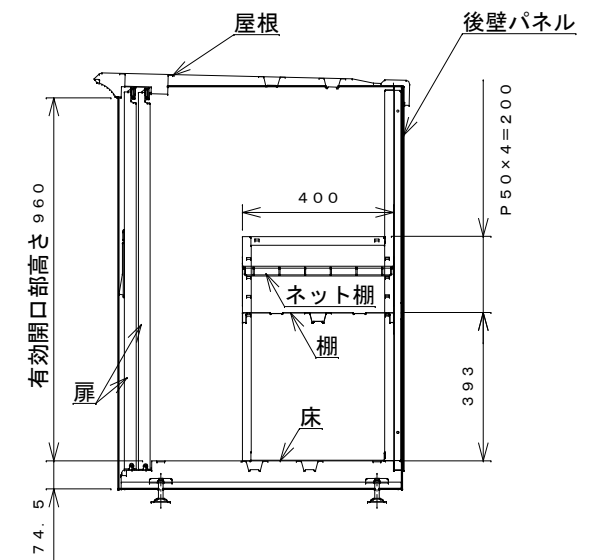
側面断面図
