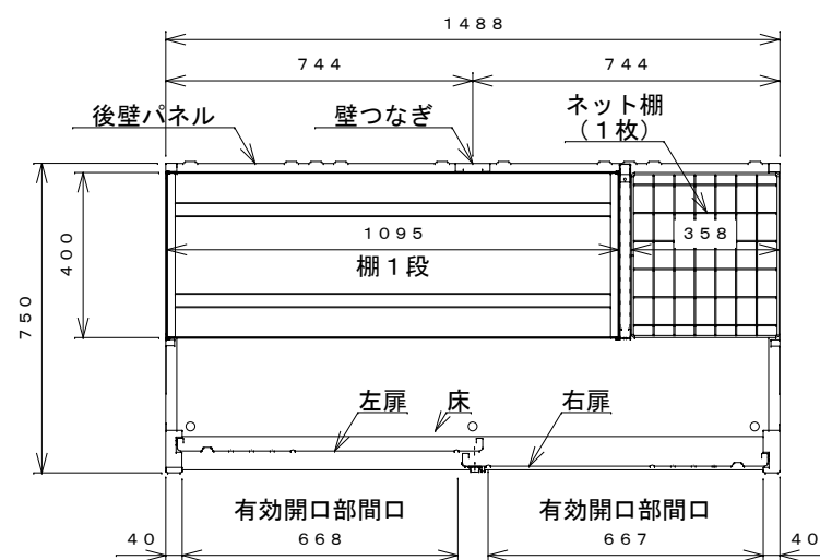
平面断面図
