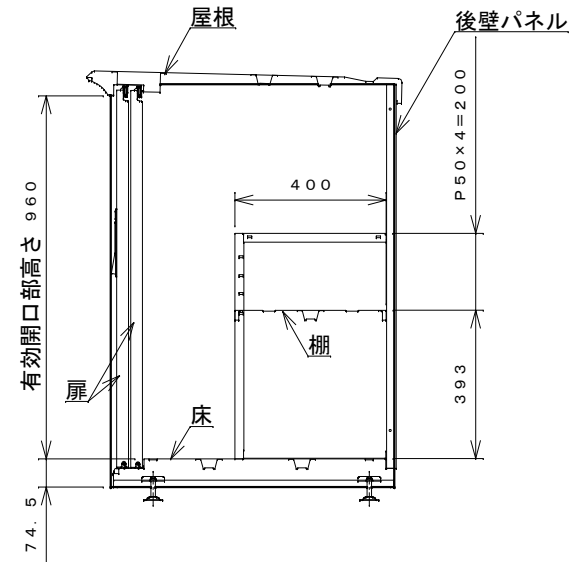
側面断面図
