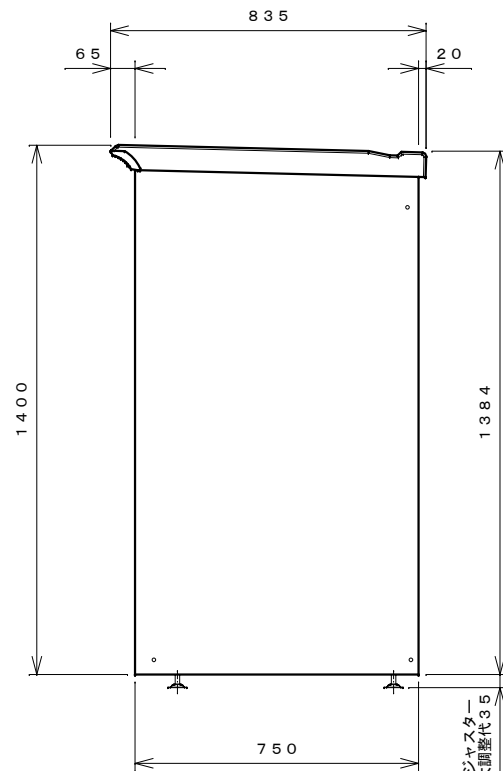
右側面図
