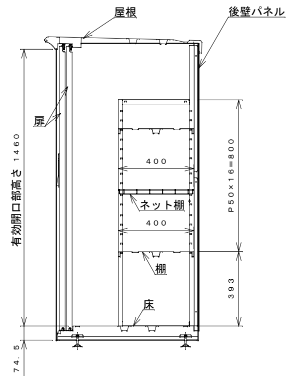
側面断面図
