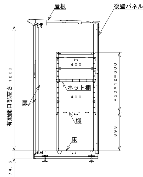
側面断面図
