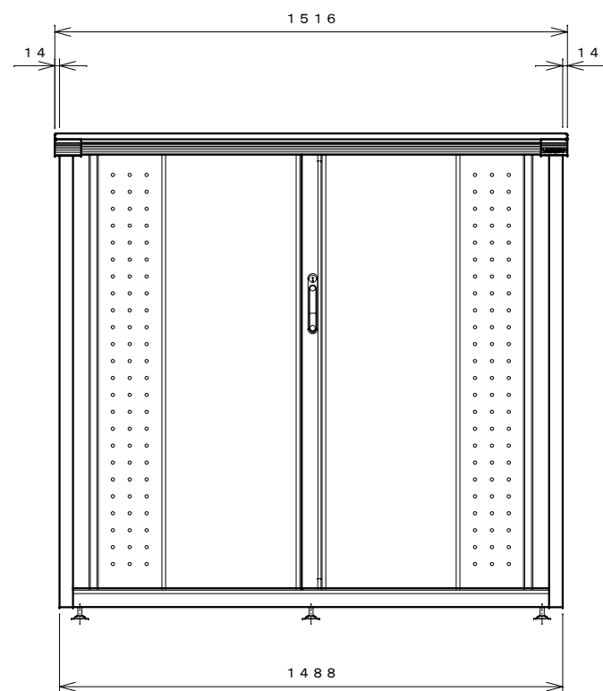
正面図
