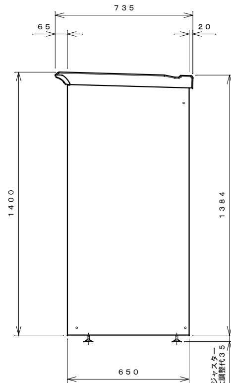
右側面図
