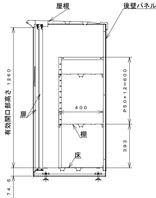
側面断面図
