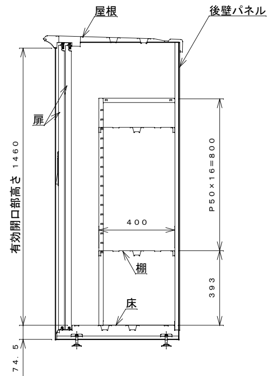
側面断面図
