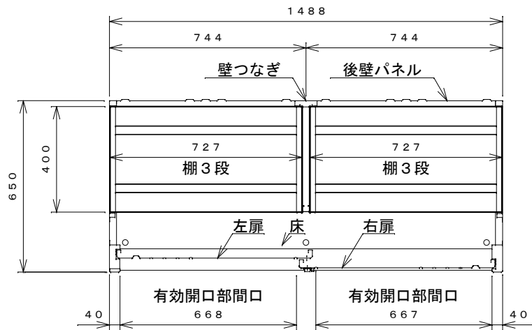
平面断面図
