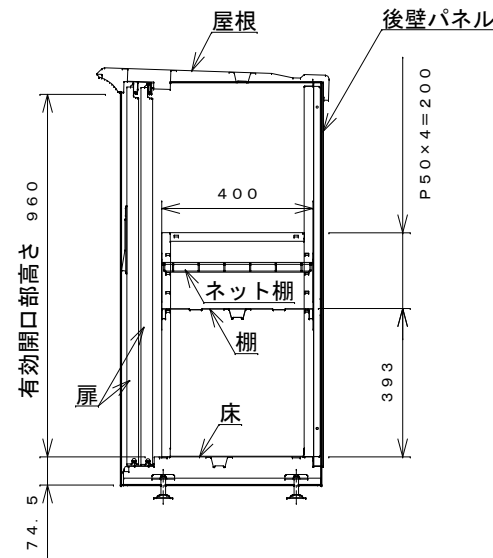
側面断面図
