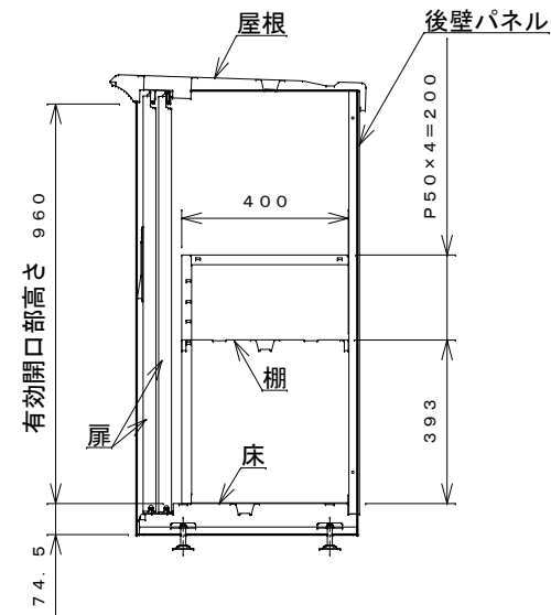
側面断面図
