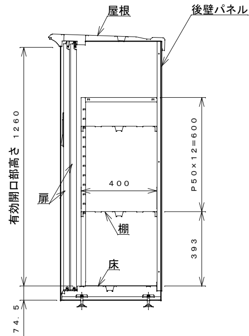
側面断面図
