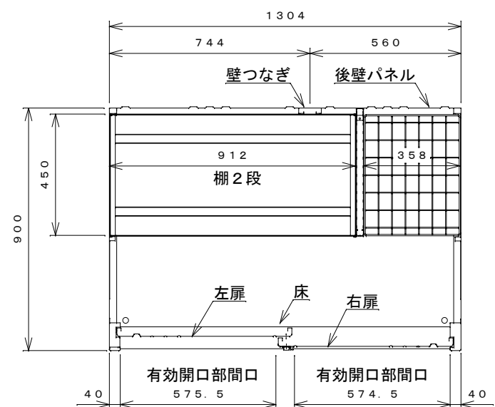
平面断面図
