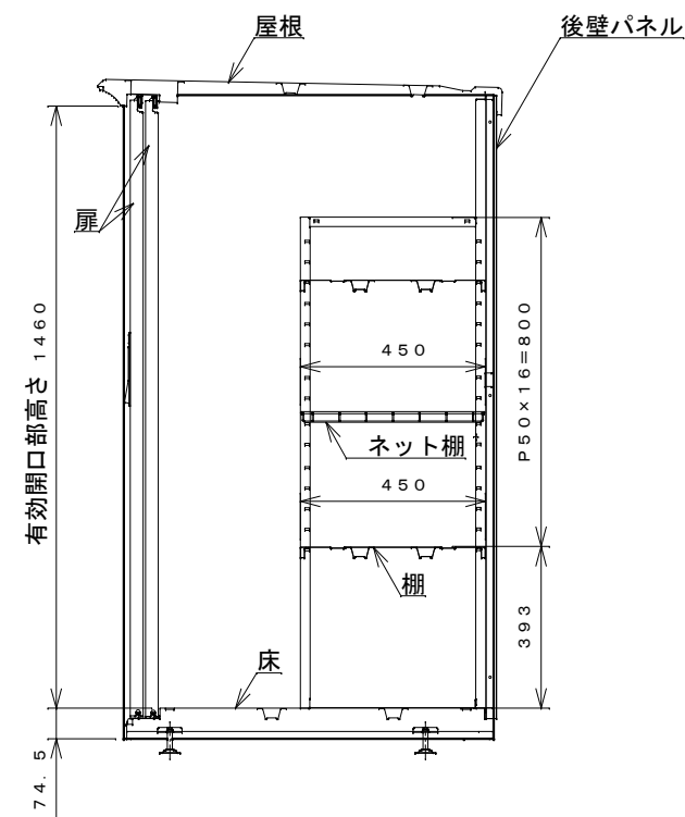
側面断面図
