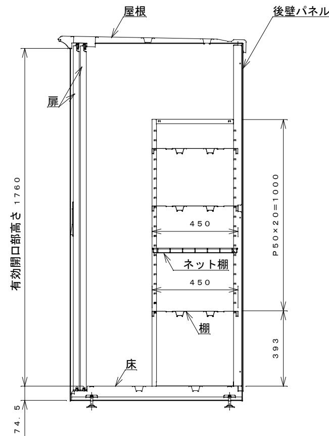
側面断面図
