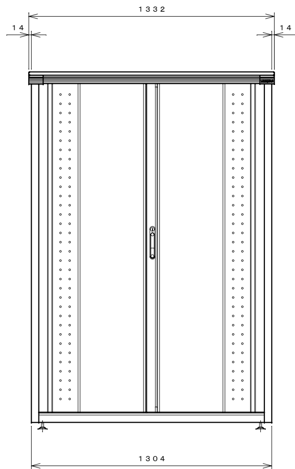
正面図
