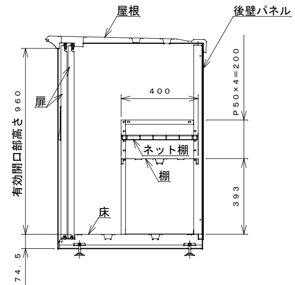
側面断面図
