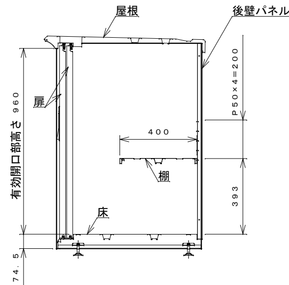
側面断面図
