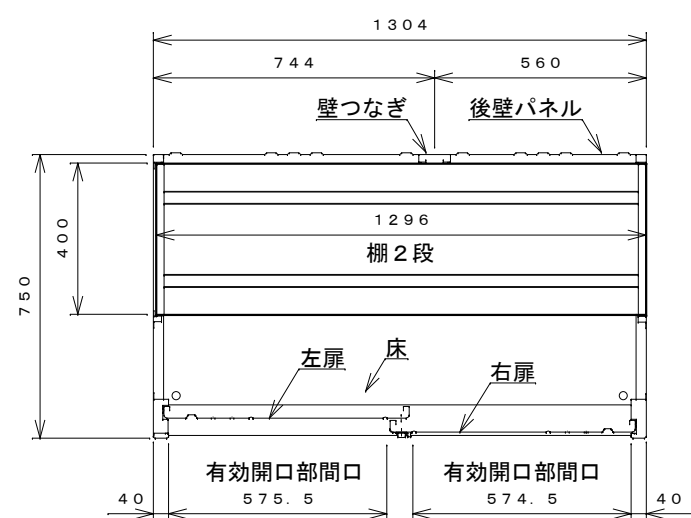
平面断面図
