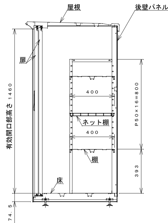
側面断面図
