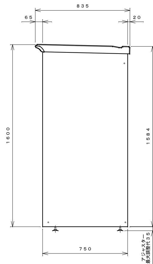
右側面図
