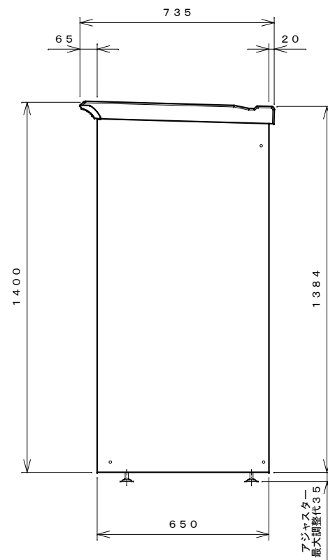
右側面図
