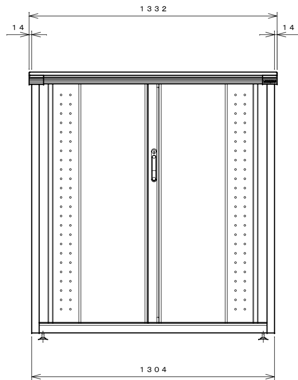
正面図
