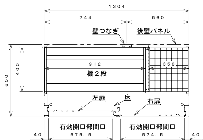
平面断面図
