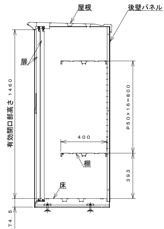
側面断面図
