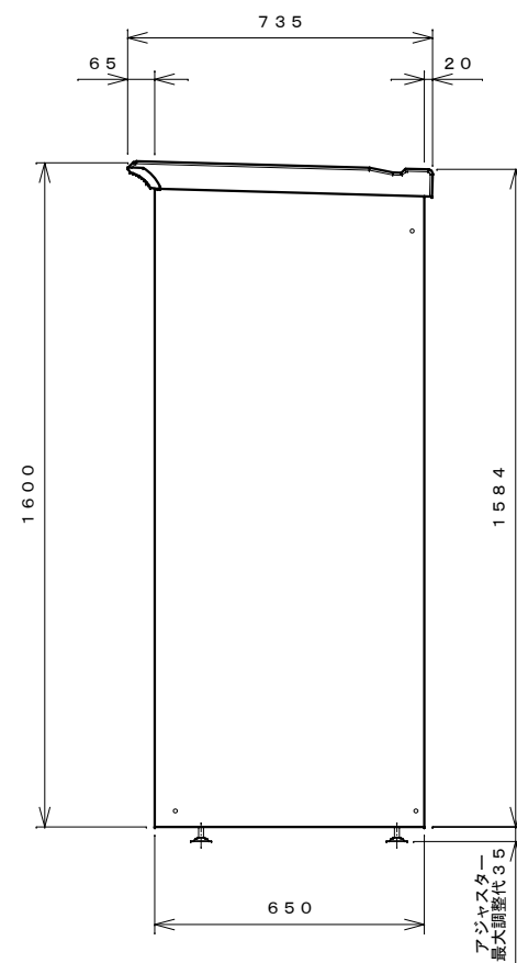
右側面図
