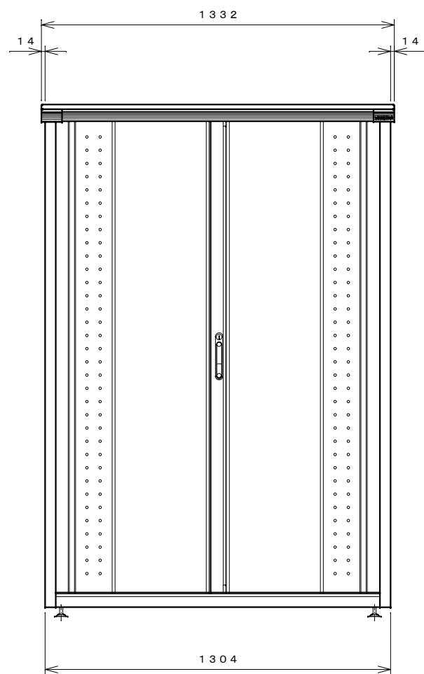
正面図
