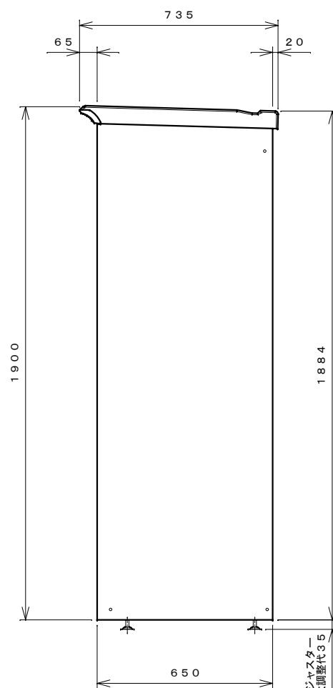
右側面図
