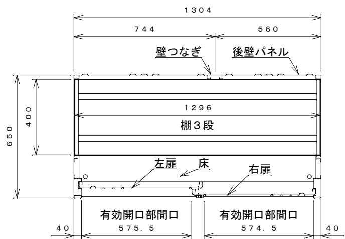
平面断面図
