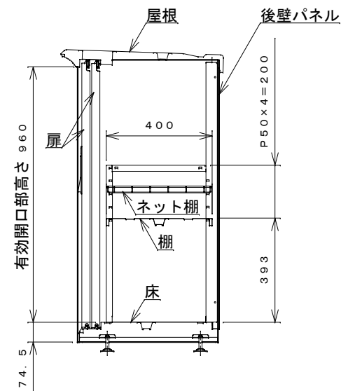
側面断面図
