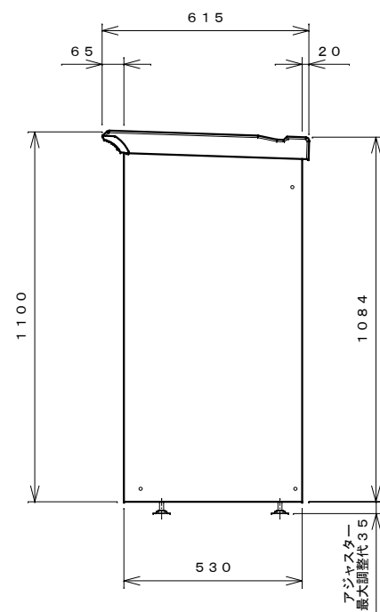
右側面図
