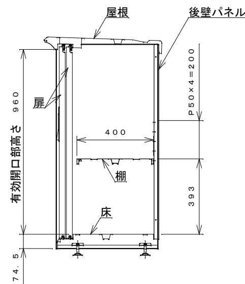
側面断面図
