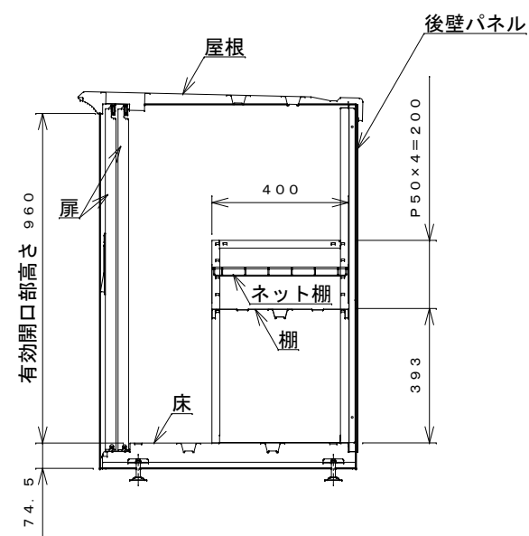
側面断面図
