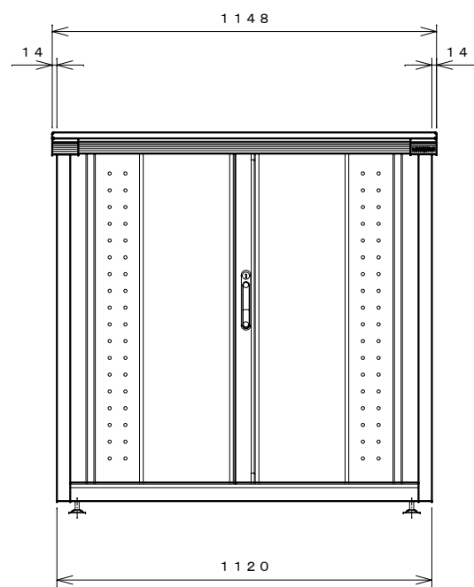
正面図
