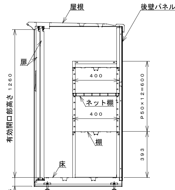
側面断面図
