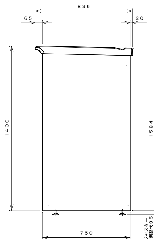
右側面図
