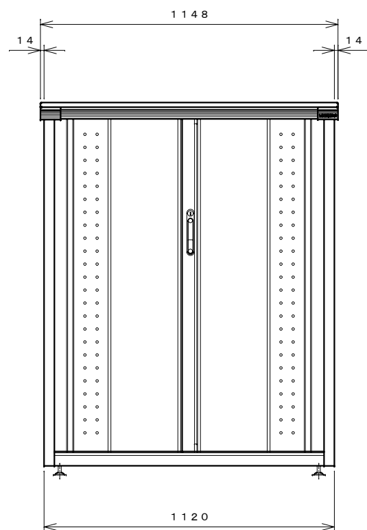
正面図
