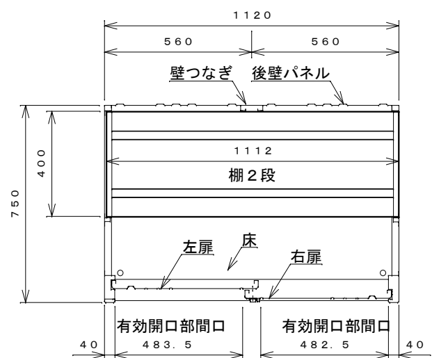
平面断面図
