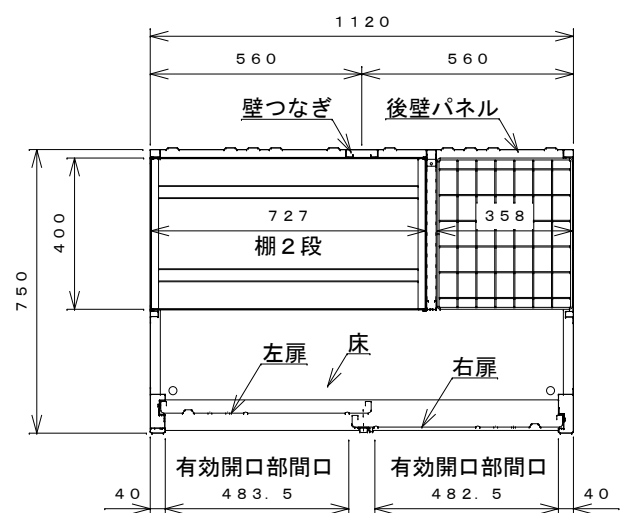
平面断面図
