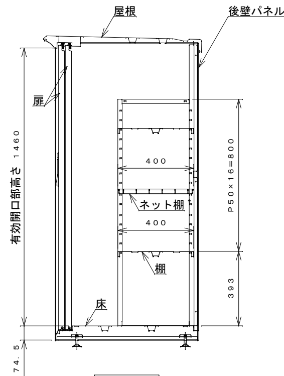
側面断面図
