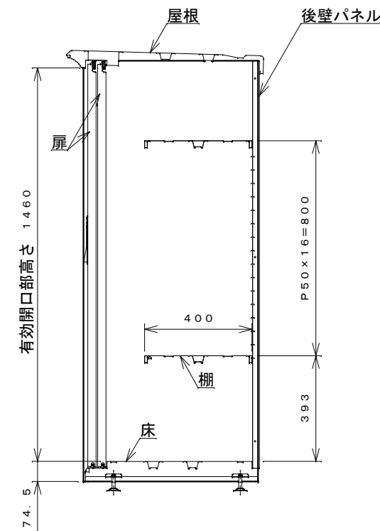
側面断面図
