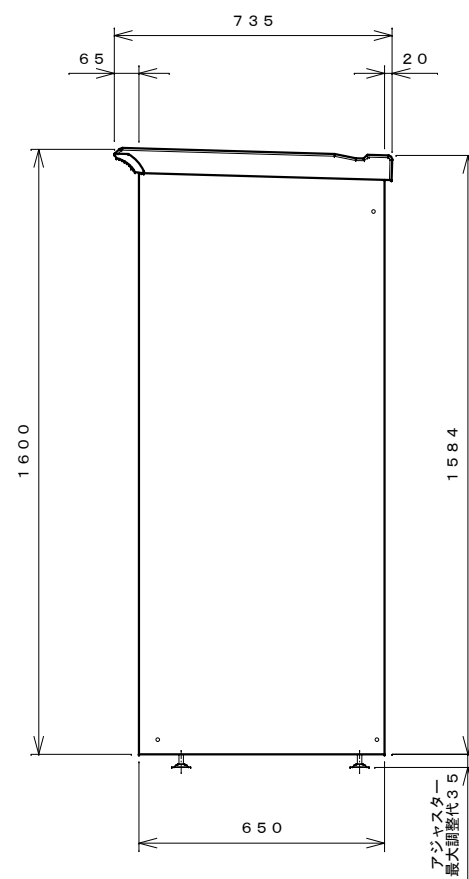
右側面図
