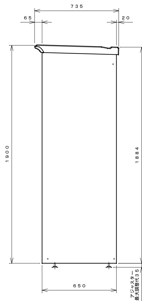
右側面図
