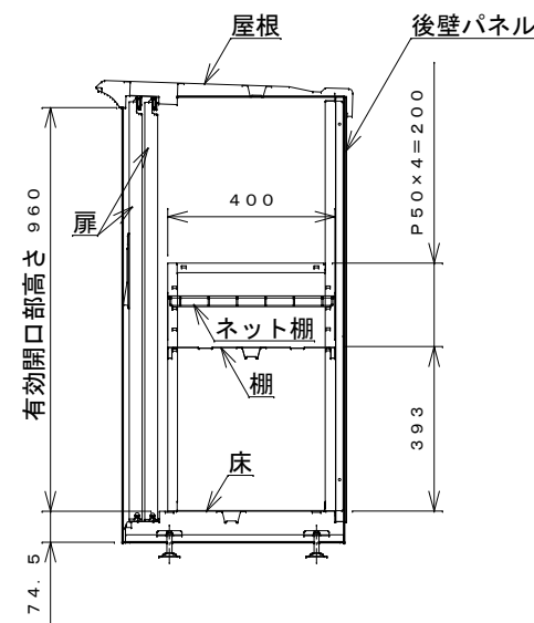
側面断面図
