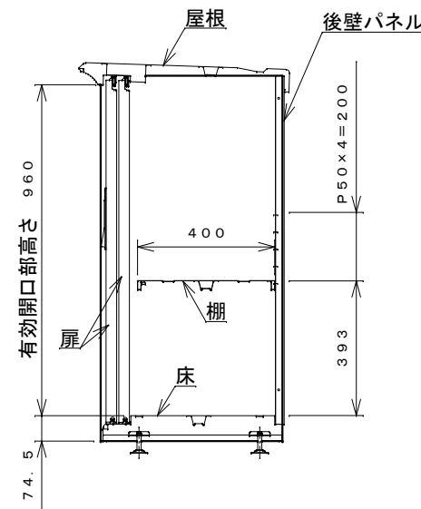
側面断面図
