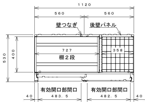
平面断面図
