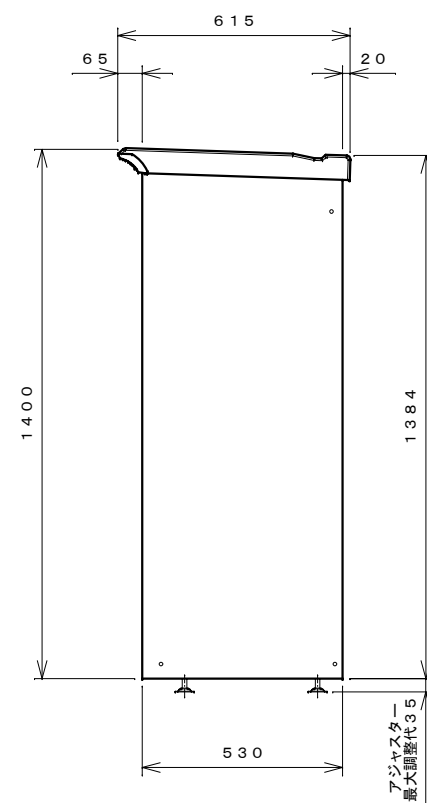
右側面図
