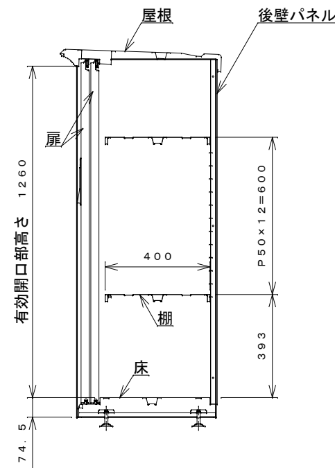
側面断面図
