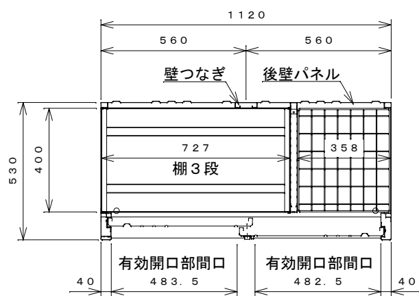
平面断面図
