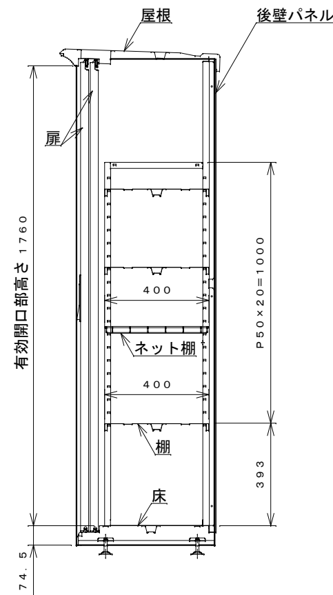
側面断面図
