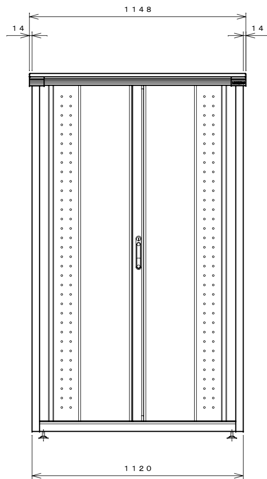
正面図
