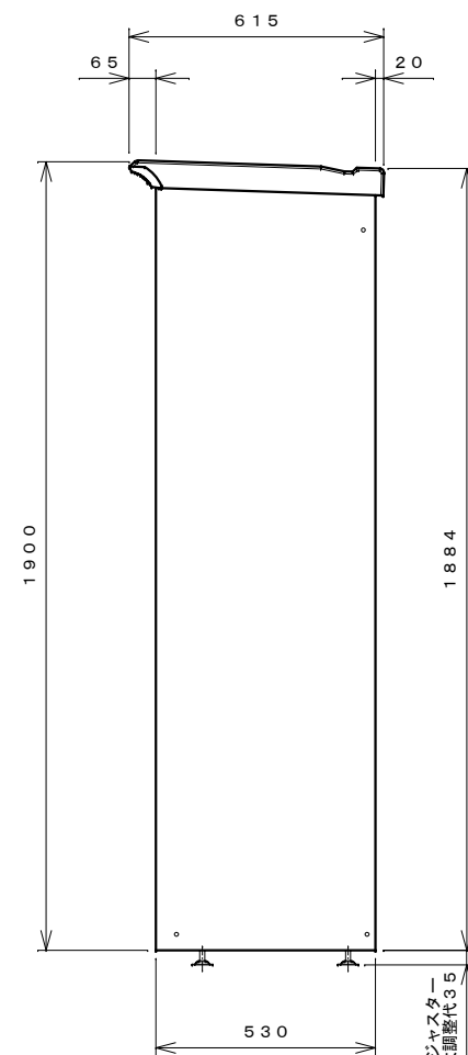
右側面図
