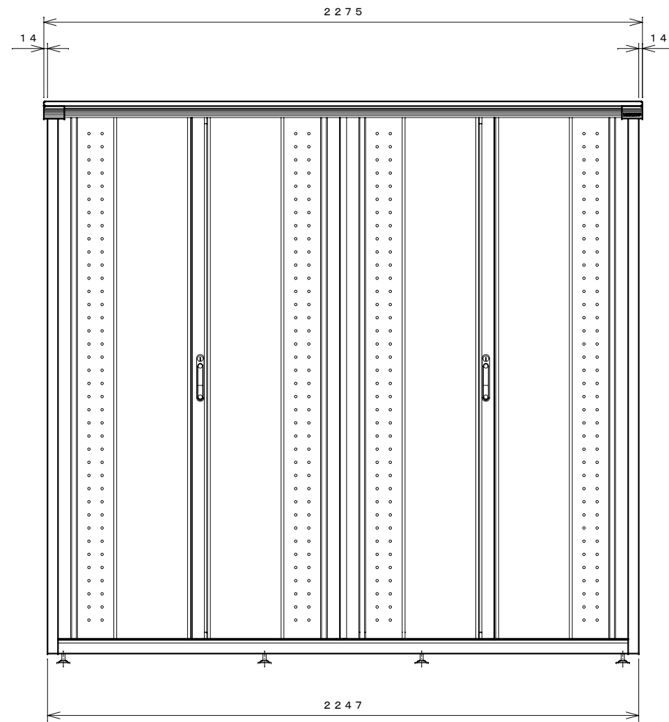
正面図
