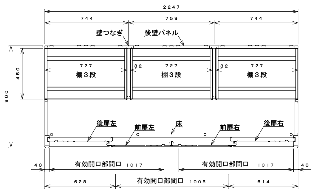
平面断面図
