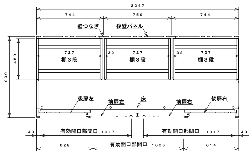
平面断面図
