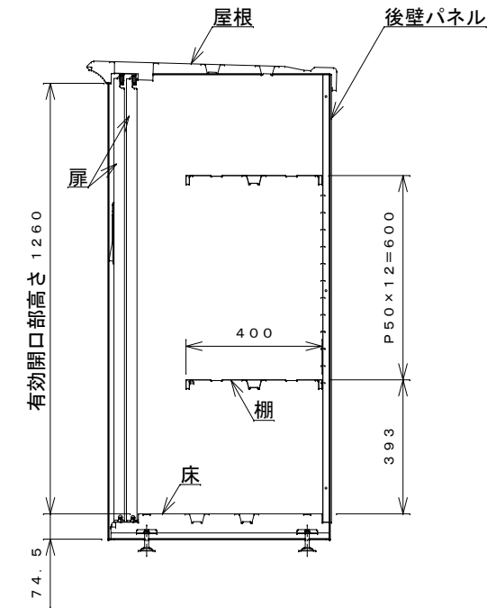
側面断面図
