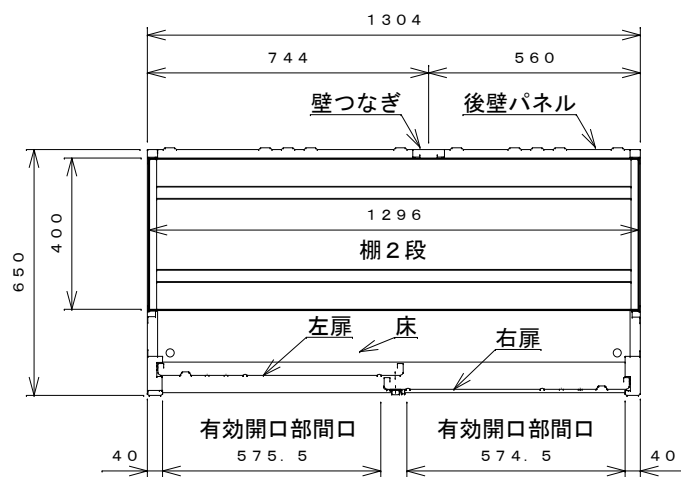
平面断面図
