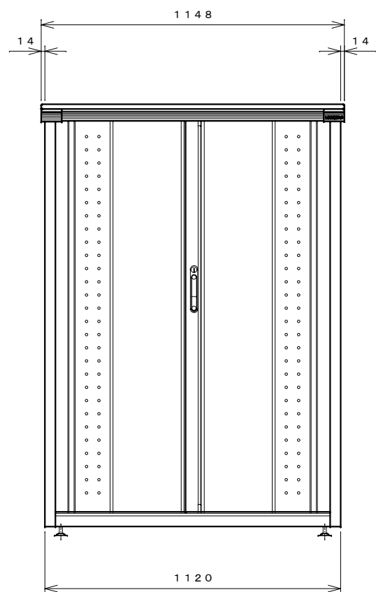
正面図
