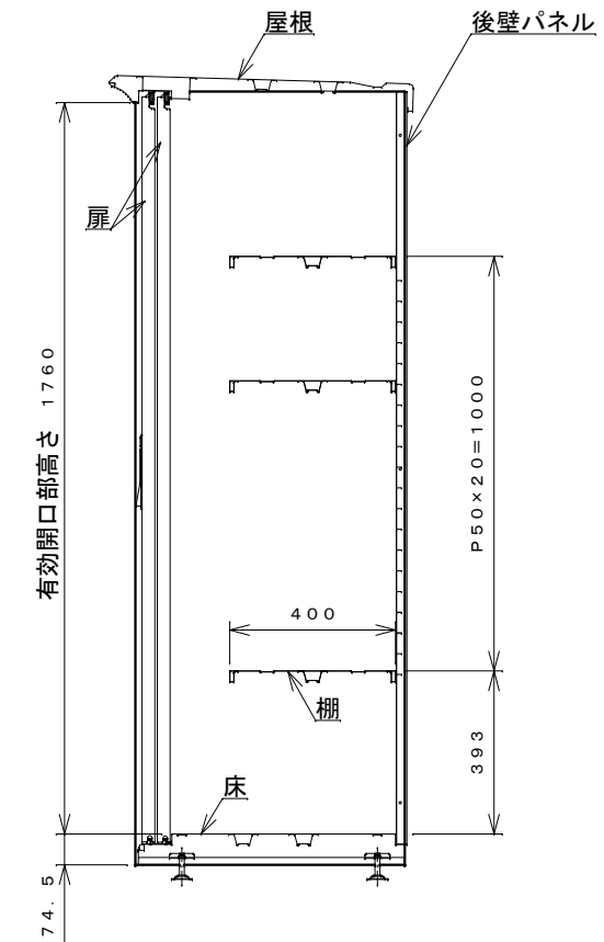
側面断面図
