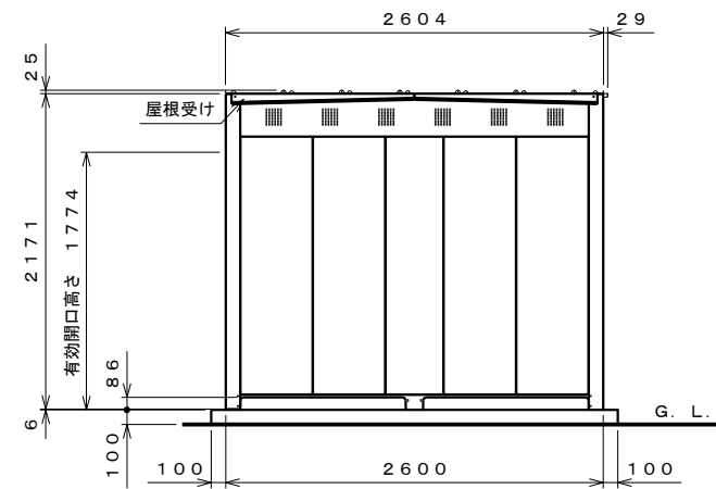
側面図 S=1:40
