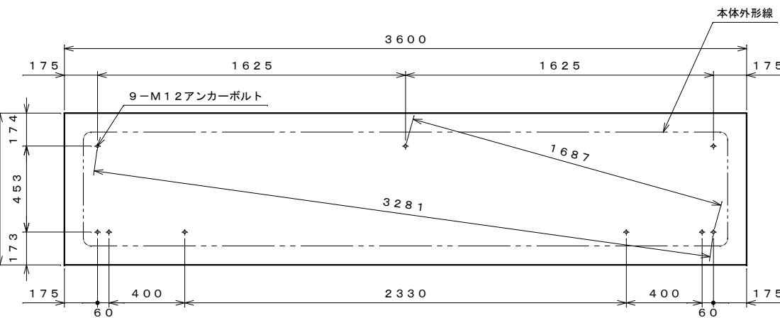
基礎伏せ図 S=1:20
