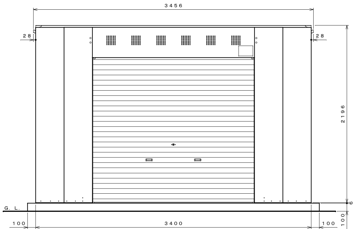
正面図 S=1:20
