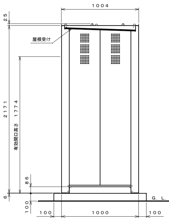
側面図 S=1:20
