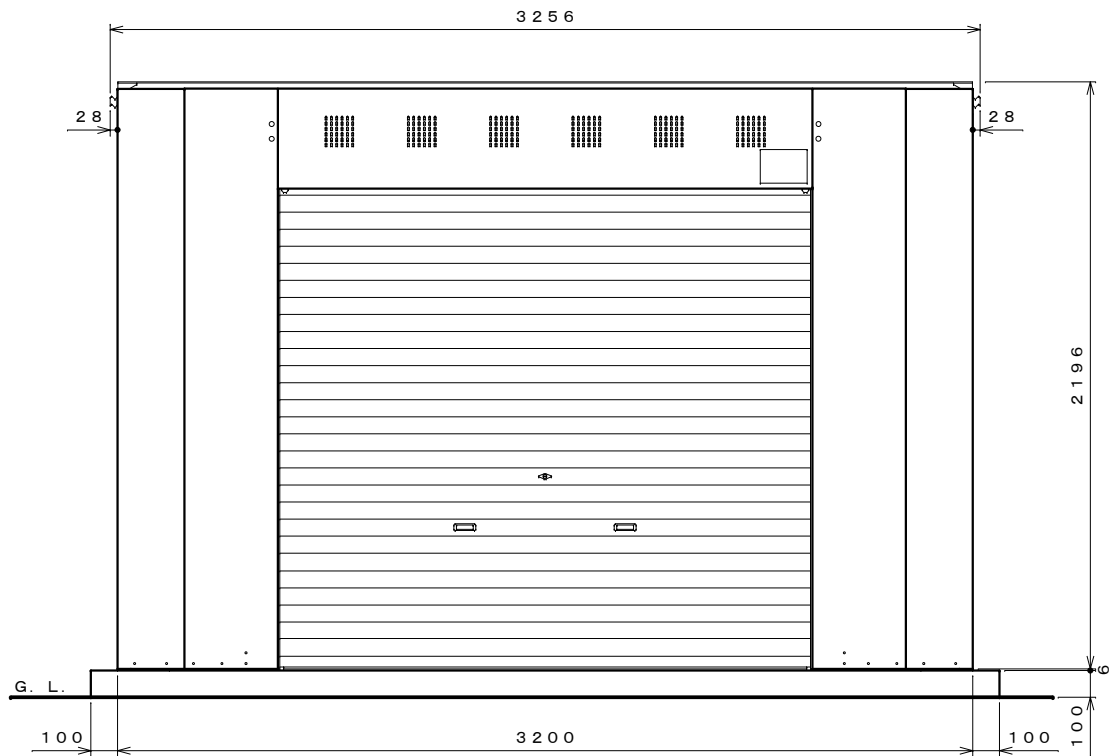
正面図 S=1:20
