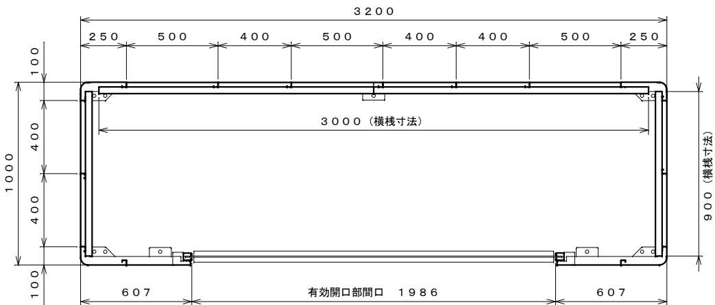
平面図 S=1:20
