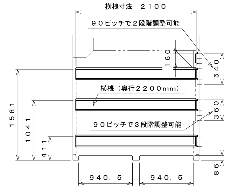
内面図 S=1:40
