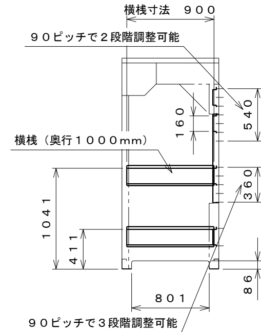
内面図 S=1:40
