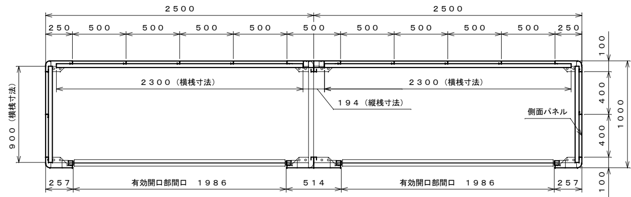
平面図 S=1:25
