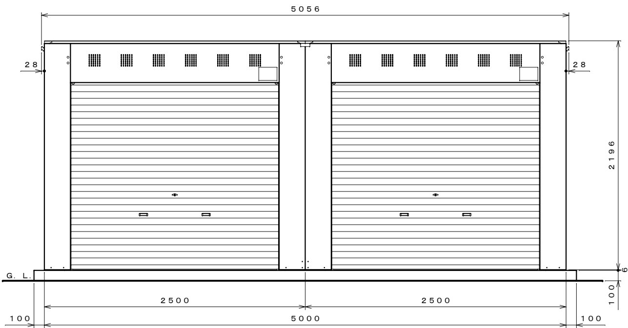
正面図 S=1:25
