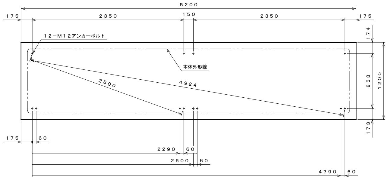
基礎伏せ図 S=1:25
